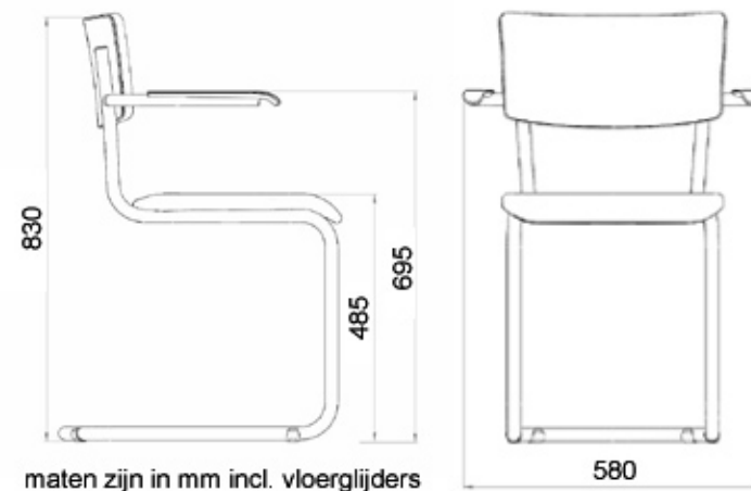
maten zijn in mm incl. vloerglijders
