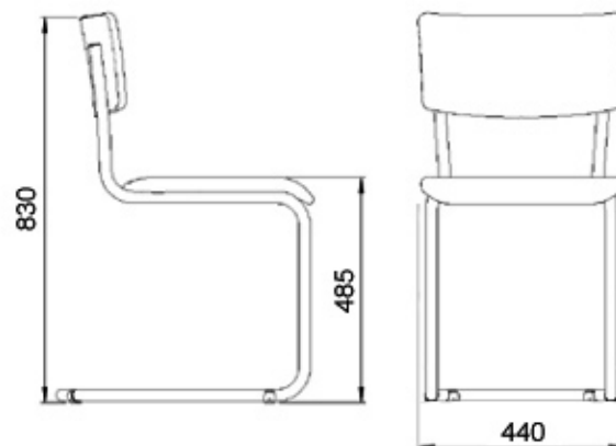
maten zijn in mm incl. vloerglijders
